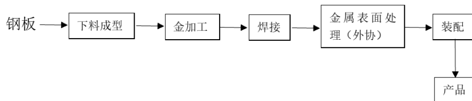
受核查方生产工艺流程图
